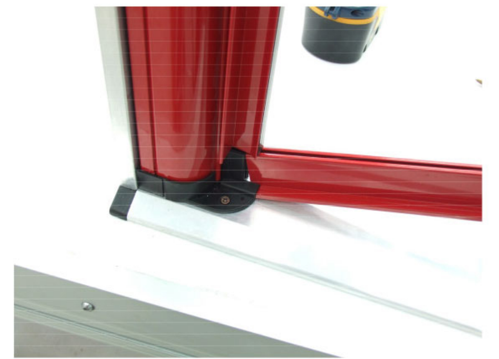
13 inserire la guida inferiore nel copri testata
