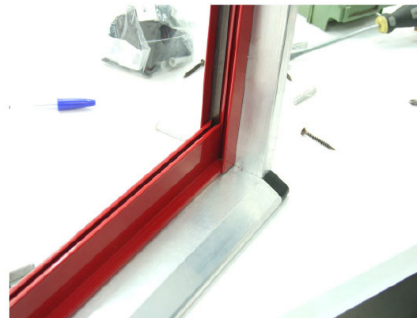
14 inserire guida inferiore nella guida laterale
