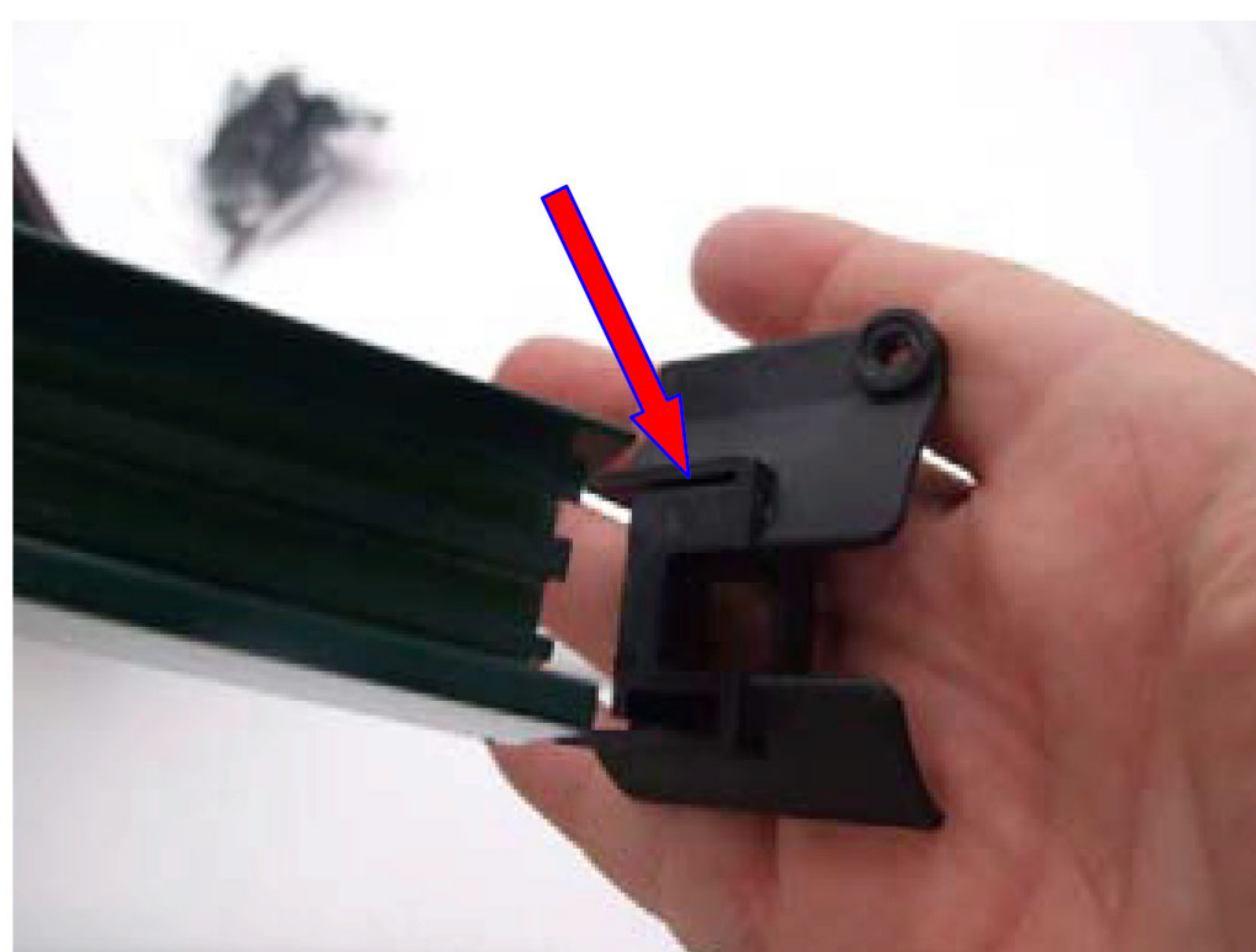
9° inserire zoccolo parte inferiore della guida
