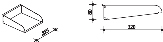
Vaschetta UNI A4 Bac UNI A4 UNI A4 tray kleine Konsole UNI A4 Bandeja UNI A4
