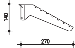
Portagrucce Porte-cintres Clothes-hanger rack Kleiderbügelträger Portaperchas
