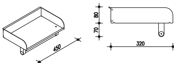
Mensola appendiabiti Etagère porte-vêtements Clothes shelf Konsole mit Kleiderstange Estante con perchero
