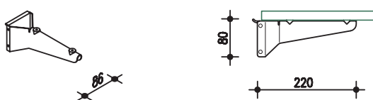
Vaschetta UNI A4 Bac UNI A4 UNI A4 tray kleine Konsole UNI A4 Bandeja UNI A4
