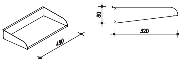
Vaschetta UNI A3 Bac UNI A3 UNI A3 tray kleine Konsole UNI A3 Bandeja UNI A3
